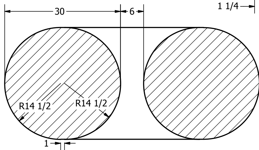
SECTION A-A SCALE 0.07 : 1
